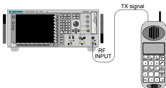
Bild 3-1 MS Messaufbau
