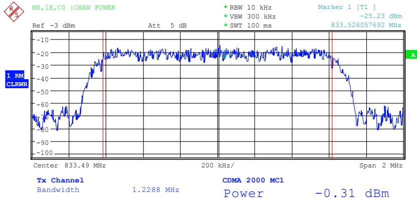
Bild 6-1 Messung der Leistung im 1.2288-MHz-Übertragungskanal
