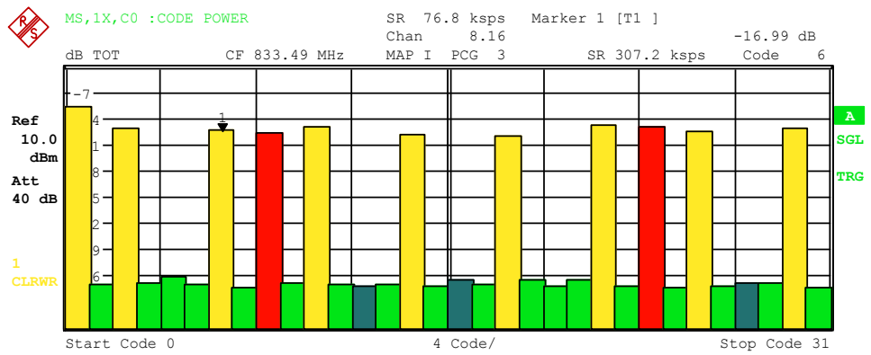
Bild 6-7 CDP-Diagramm in Hadamard-Ordnung
