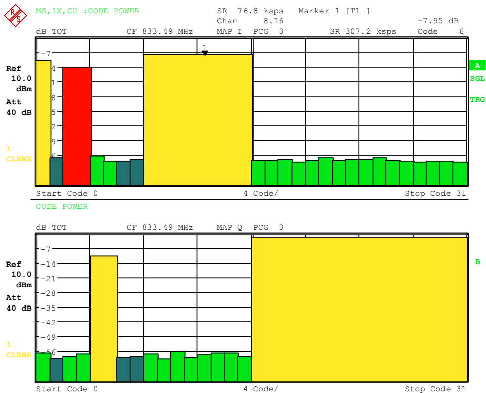
Bild 6-9 CDP-Diagramm in BitReverse-Ordnung im Überblicksmodus
