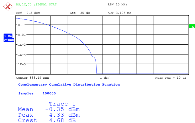
Bild 6-5 CCDF des cdma2000–Signals
