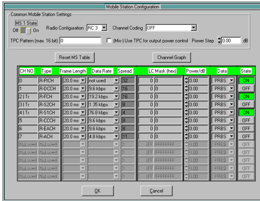
Bild 2-2 WinIQSIM – Konfiguration mit aktiven Kanälen
